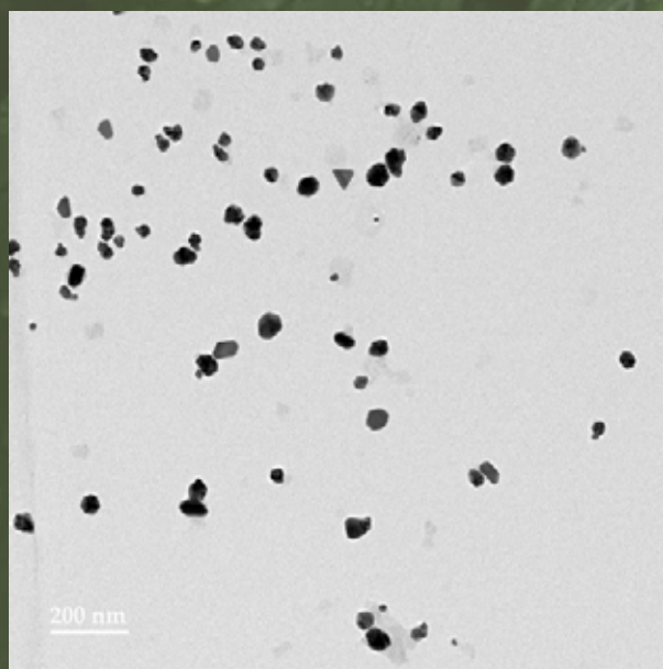
TEM Image of USK-AG-00111
